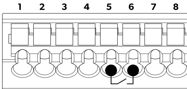
Pillanatkapcsoló csatlakoztatása ( . ábra 5 268. oldal ,5)
