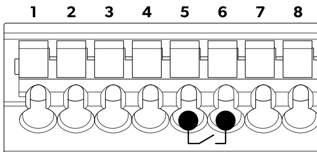
Anslutning av externt impulsdon ( bild. 5 sida 159,5)
