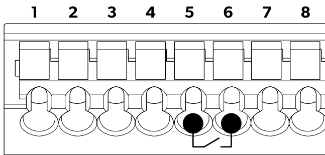
Priključitev momentnega stikala (📷 sl. 5 na strani 322, 5)
