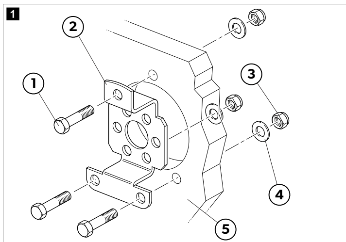
90° brakett
