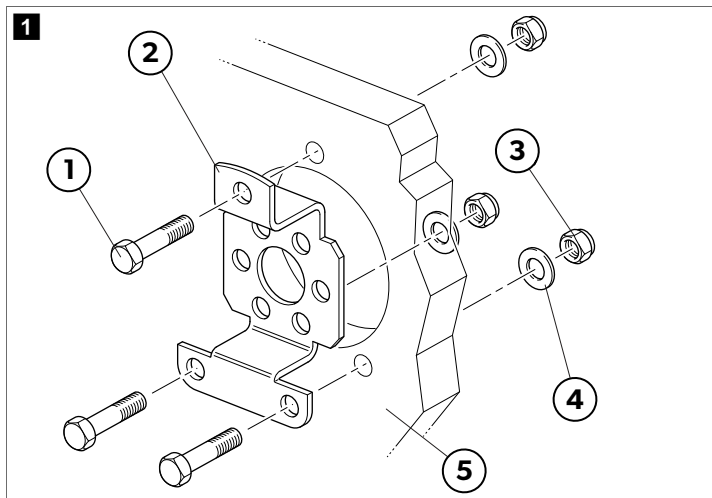
Nosač od 90°
