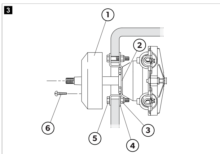
SH5150-roer afgebeeld
