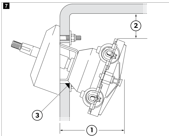
Rama 20° (na ilustracji model SH5150)
