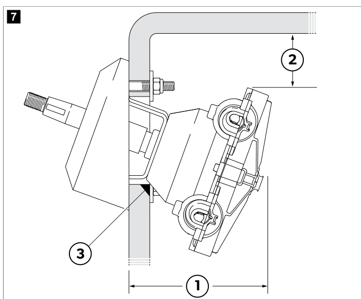
Ramă la 20° (SH5150 în imagine)
