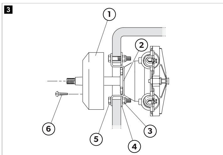
Lenkgetriebe SH5150 abgebildet
