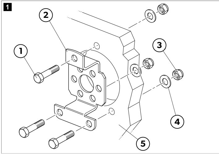
90° braket
