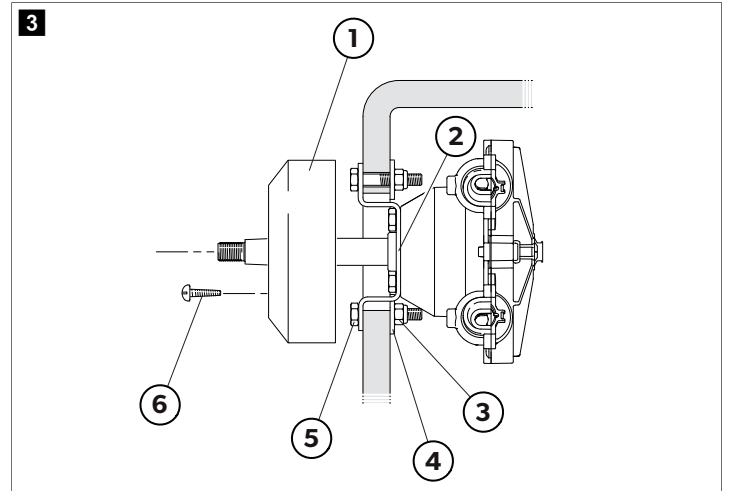
SH5150 Dümen gösterilmiştir
