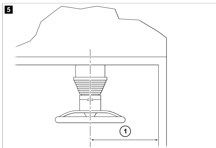
Aro de 20° (SH5150 apresentado)
