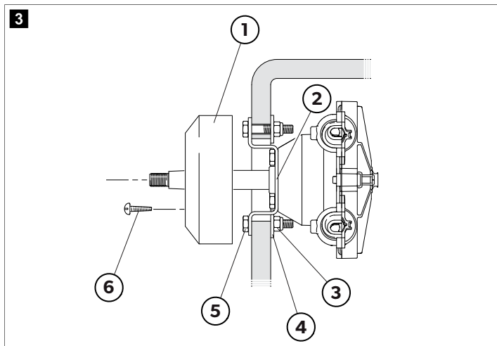
Näidatud on rool SH5150
