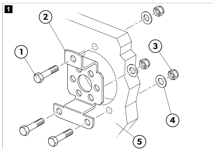
90° držák
