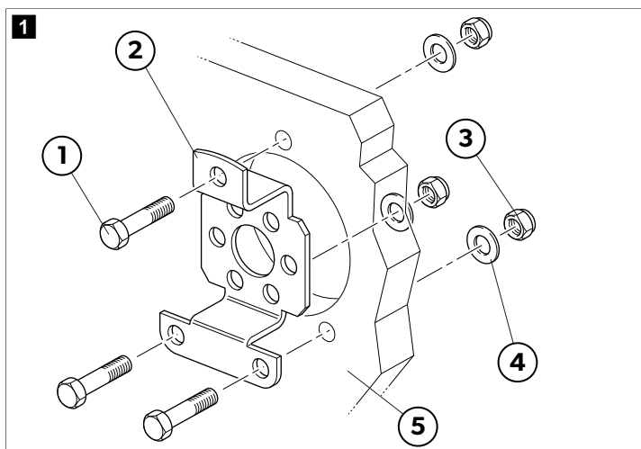
Consolă la 90°
