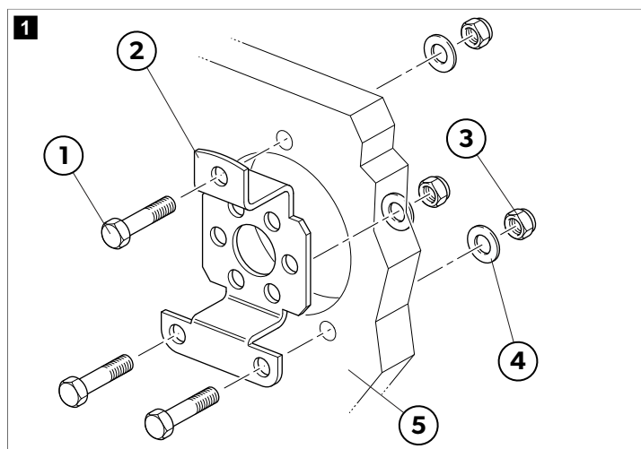
90° kronšteins
