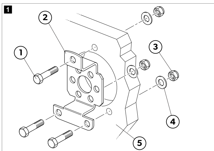
Suporte de 90°
