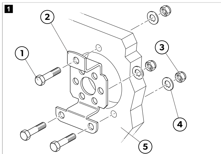
90 ° Halterung
