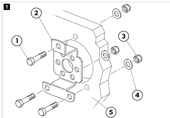
90° konzola
